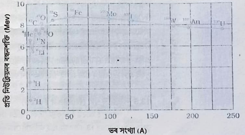
চিত্ৰ 13.1 প্ৰতিনিউক্লিয়নৰ বন্ধন শক্তিৰ ভবসংখ্যাৰ ফলন হিচাপে দেখুওৱা হৈছে।
