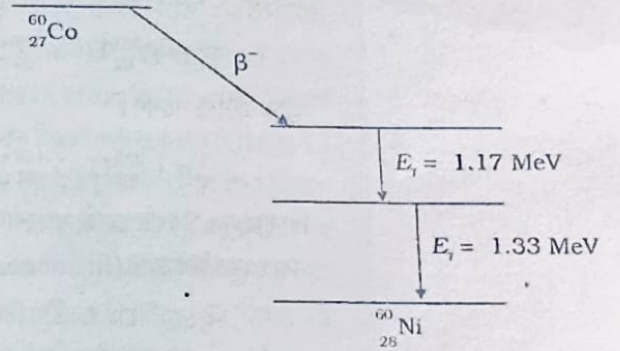
চিত্ৰ 13.4 {}_{27}^{60}\text{Co} নিউক্লিয়াছৰ বিটা বিঘটনৰ পাছত হোৱা \gamma ৰশ্মি নিৰ্গমনৰ শক্তিস্তৰ চিত্ৰ।
