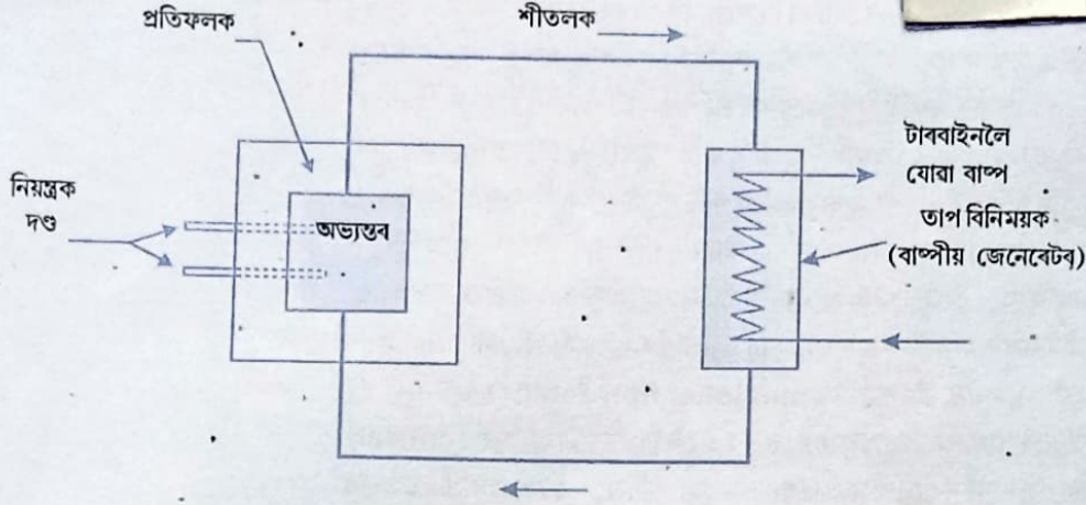
চিত্র 13.5 তাপীয় নিউট্রনৰ দ্বাৰা সংঘটিত বিয়োজন ভিত্তিক নিউক্লীয় বিএক্টৰৰ আঁচনি চিত্র।
