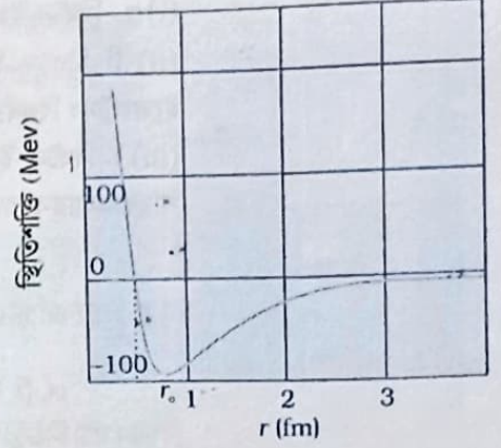
চিত্ৰ 13.2 এযোৰ নিউক্লিয়নৰ স্থিতিশক্তিক সিহঁতৰ মাজৰ ব্যৱধানৰ ফলন হিচাপে দেখুওৱা হৈছে। r_0 তকৈ বেছি ব্যৱধানত আকৰ্ষণ হয় আৰু r_0 তকৈ কম ব্যৱধানত প্ৰবল বিকৰ্ষণ হয়।
