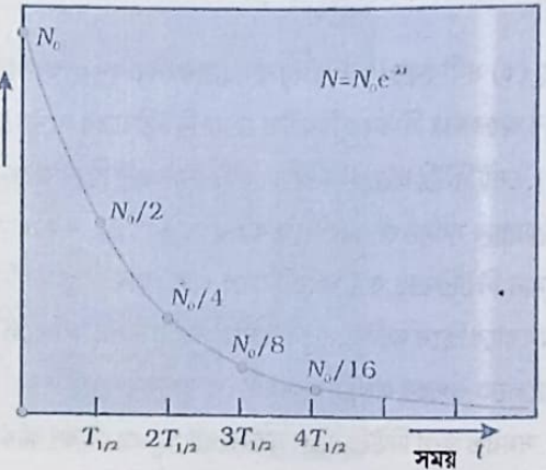
চিত্ৰ 13.3 তেজস্ক্ৰিয় নমুনা এটাৰ সূচকীয় বিঘটন। T_{1/2} সময়ত পাছত সেই নমুনাটোৰ নিউক্লিয়াছৰ সংখ্যা আধা হয়গৈ।
